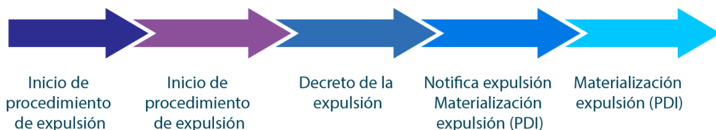
Figura 3. Flujo del proceso sancionatorio de expulsión administrativa en Chile.
